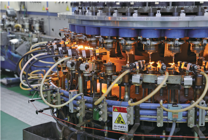
双峰格雷海姆生产线 范昀 摄
