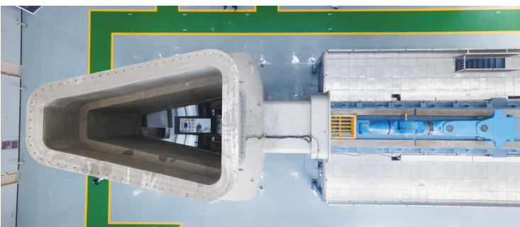
聚变堆主机关键系统综合研究设施八分之一真空室及总体安装系统主体平台 新华社发
